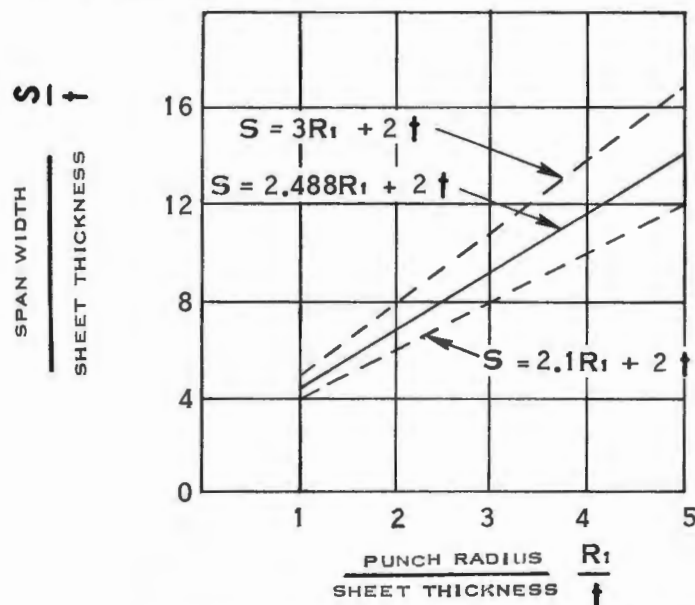
GRAPHICAL DIE OPENING VALUES FIG. 1 A-2
