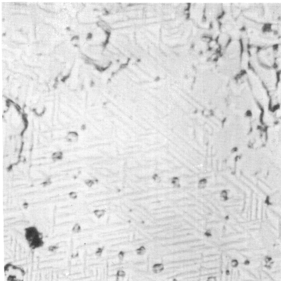
Neg. No. 3643 X800 60 glycerine, 20HNO 3 , 20HF
