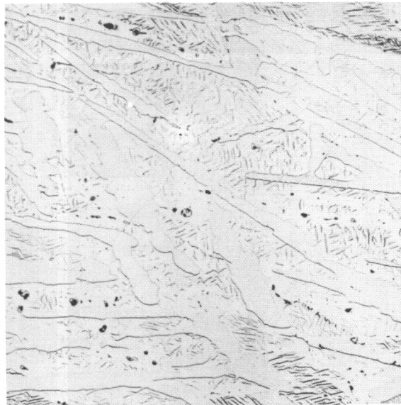
Neg. No. 3346 X250 60 glycerine, 20HNO 3 , 20HF
