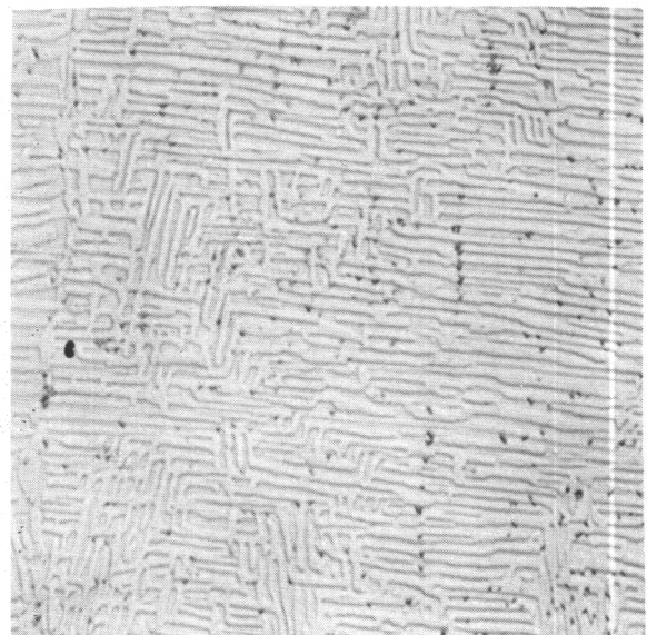
Neg. No. 3642 X800 60 glycerine, 20HNO 3 , 20HF
