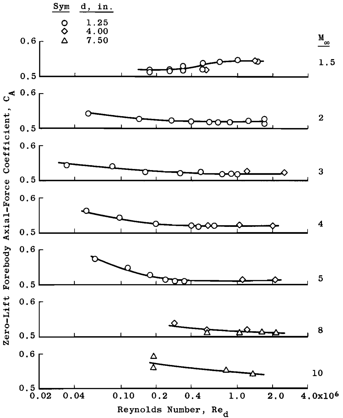
a. Configuration HB-1
