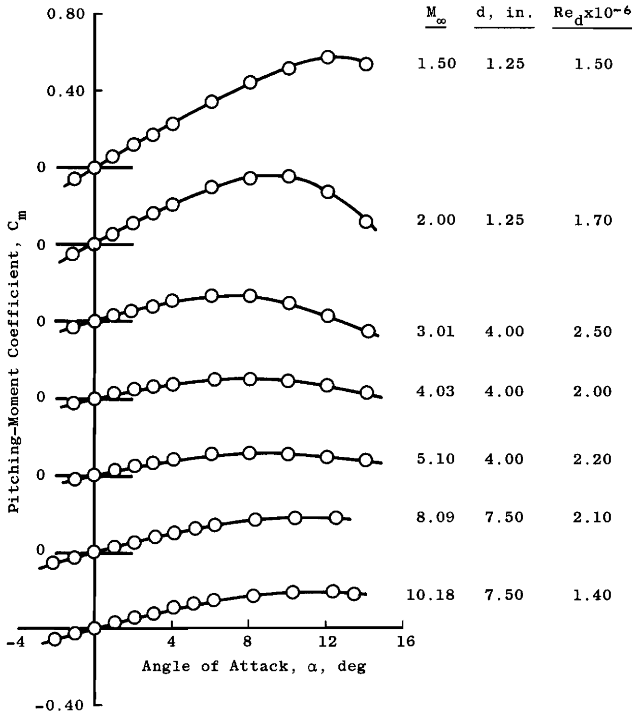
a. Configuration HB-1
